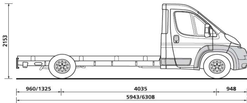
SASIU CABINA SIMPLA L3/L4
