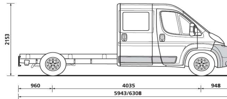
SASIU CABINA DUBLA L3
